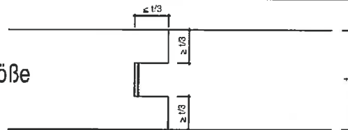
Konstruktionsbeispiel einer Deckentafel mit schubsteif verbundenen Bretterstößen
